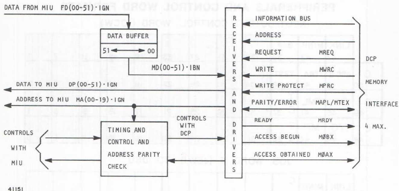
Figure IV-2-6. DCI Unit
