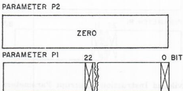
Interval Timer Interrupt Parameters
