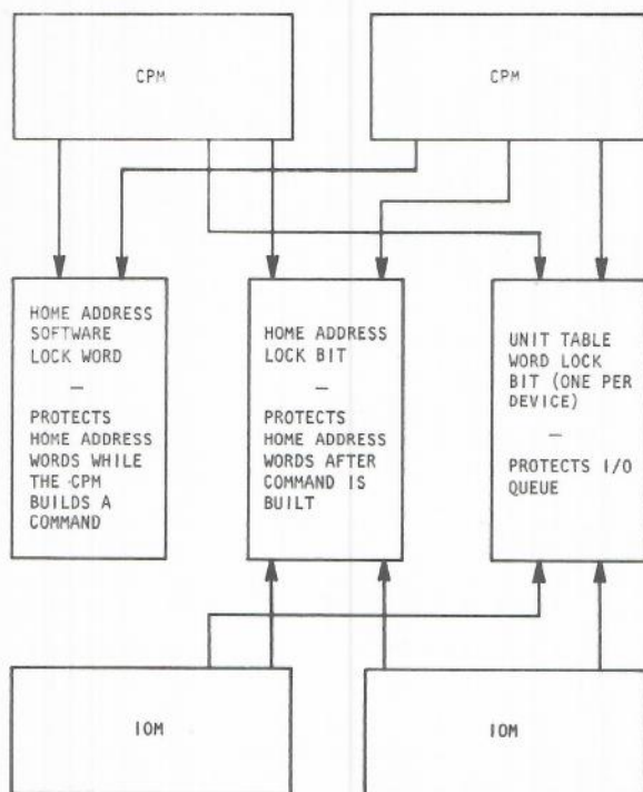
Figure II-4-4. I/O Subsystem Map Protection
